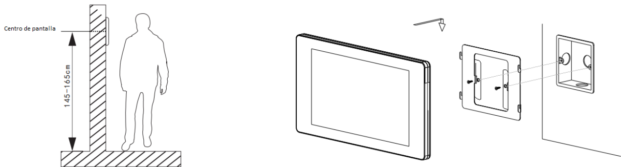
Ilustración 5: Proceso de instalación
