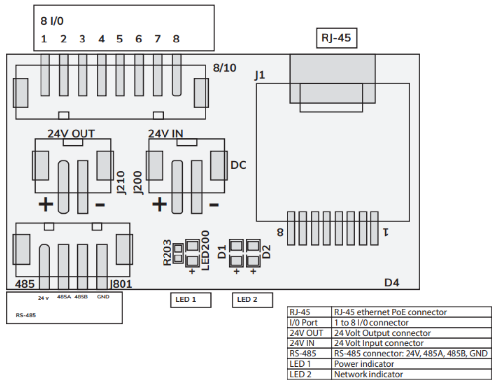
Ilustración 4: Panel de conexionado
